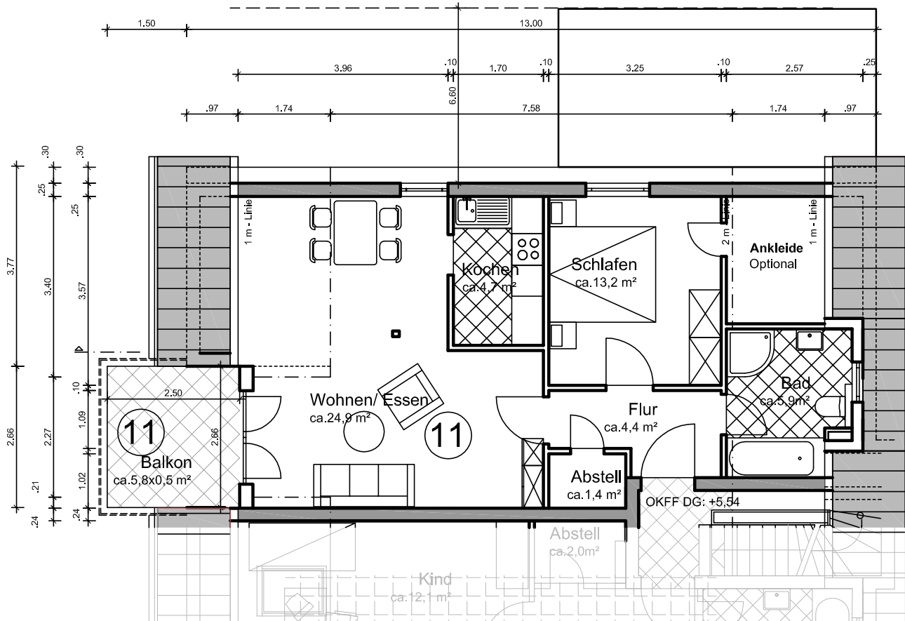
Dachgeschoss 1:100
