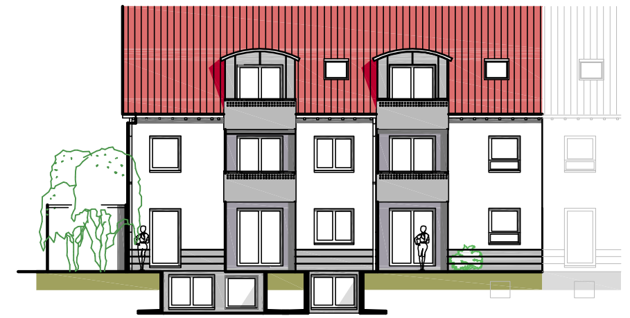
Westansicht
