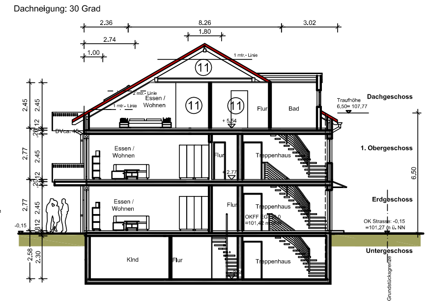
Schnitt
